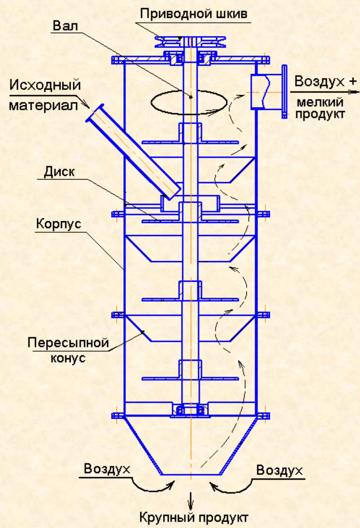
Классификатор для сортировки сыпучих материалов
