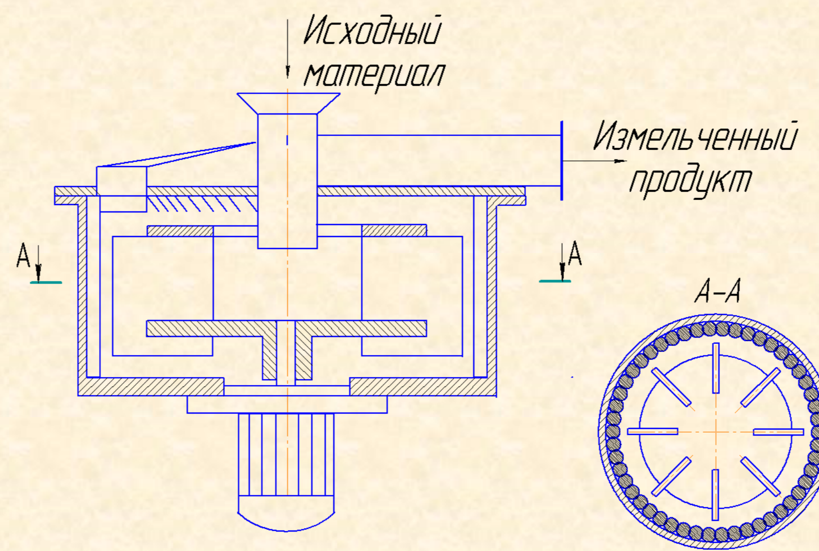
Роторно-центробежная мельница
