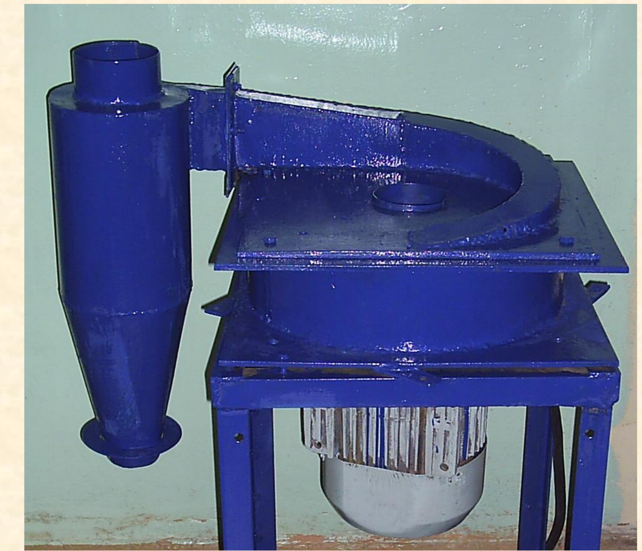
Роторно-центробежная мельница
